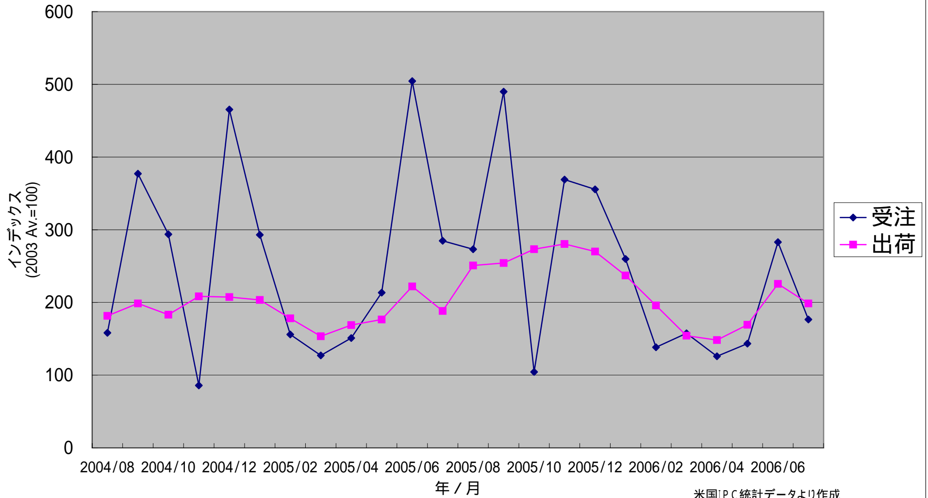
米国フレキシブルプリント配線板受注・出荷インデックス(2003 Av.=100)
